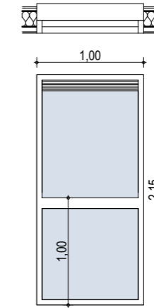
EM4 - Ensemble menuisé aluminium Teinte RAL Blanc 9010 laqué Quantité : 2 Localisation : Circulation
