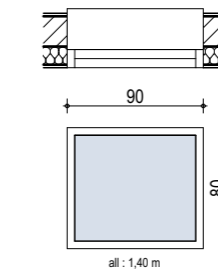
EM5 - Châssis fixe aluminium Teinte RAL Blanc 9010 laqué Quantité : 2 Localisation : Circulation
