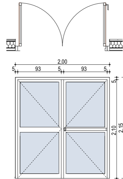
EM2 - Ensemble menuisé aluminium Teinte RAL Blanc 9010 laqué Quantité : 1 Localisation : Circulation
