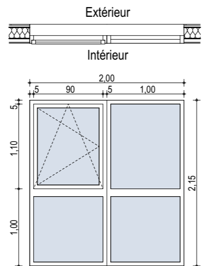
EM3 - Ensemble menuisé aluminium Teinte RAL Blanc 9010 laqué Quantité : 1 Localisation : Circulation
