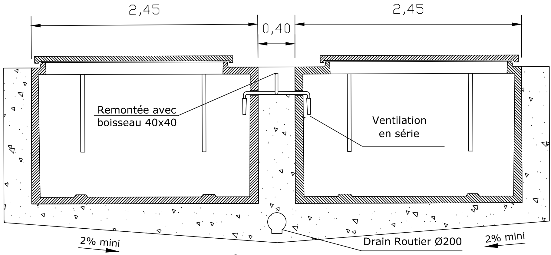
Coupe caveaux
